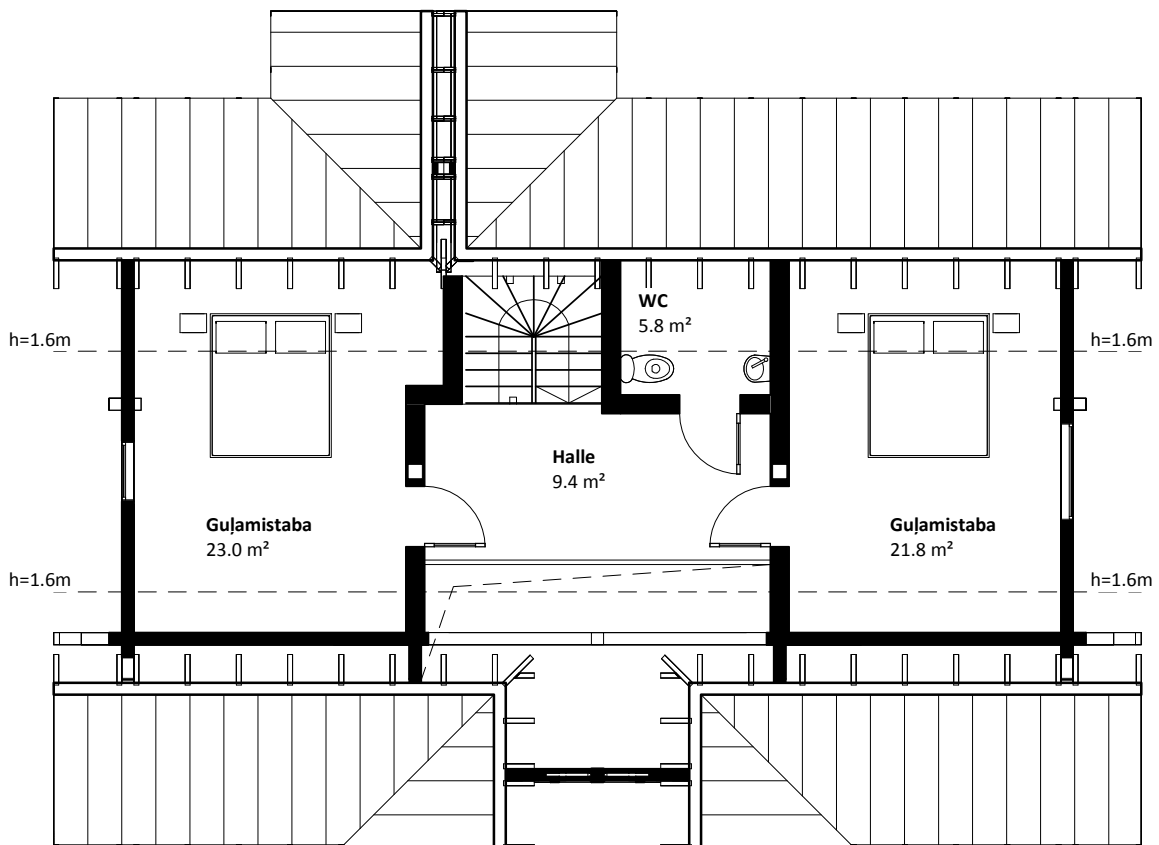
1. stāva plāns
